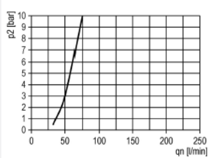
Öleransprechgrenze
